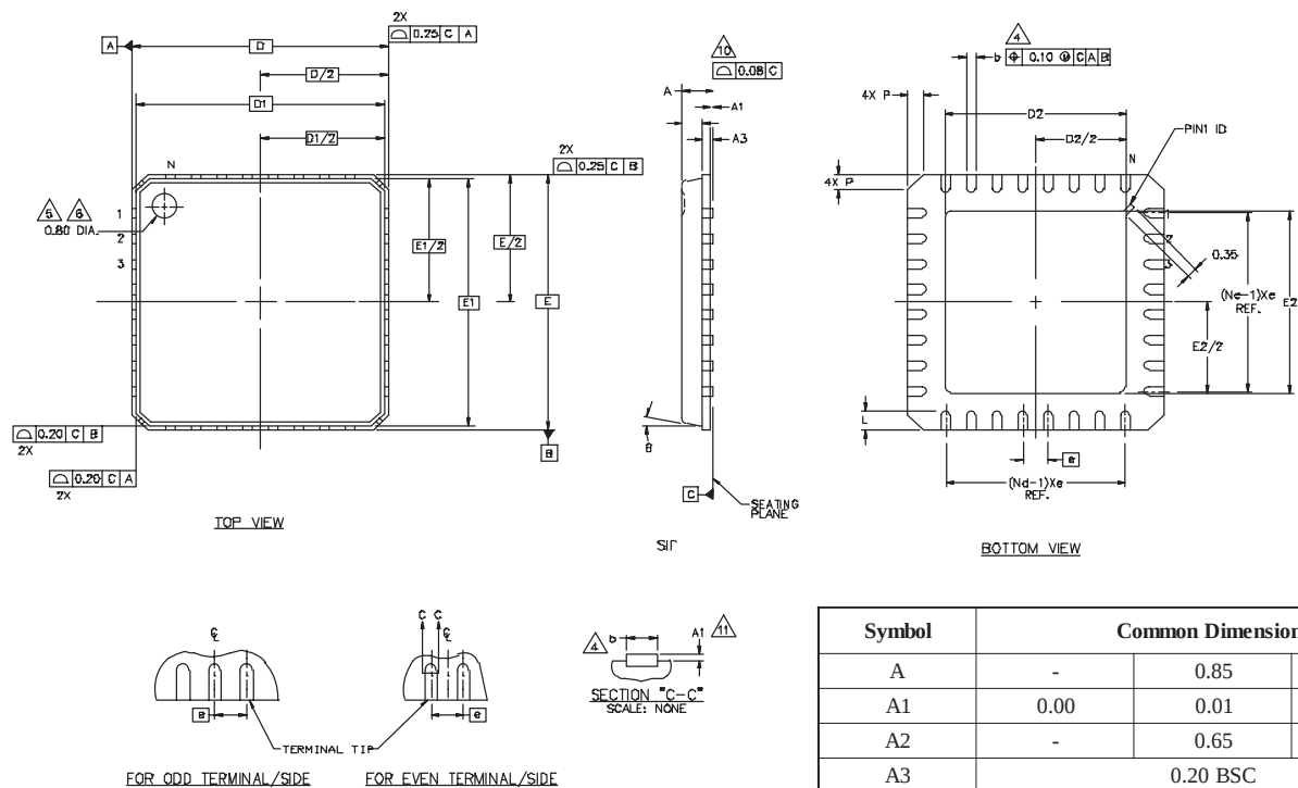
56 pin MLF2
