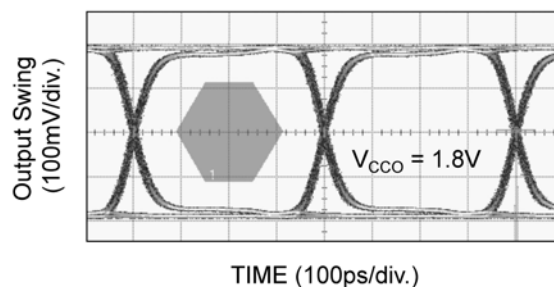
2.5Gbps Data
