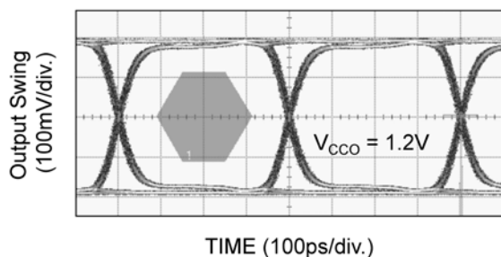
2.5Gbps Data
