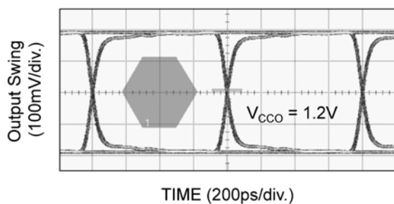
1.25Gbps Data
