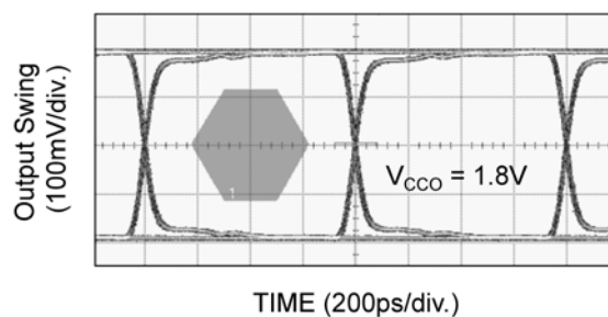
1.25Gbps Data
