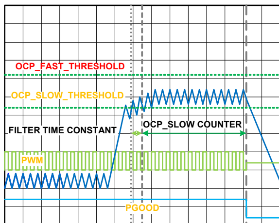
FIGURE 20. OCP_SLOW
