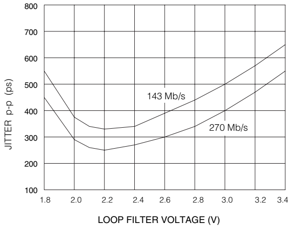
Fig. 16 Output Jitter
