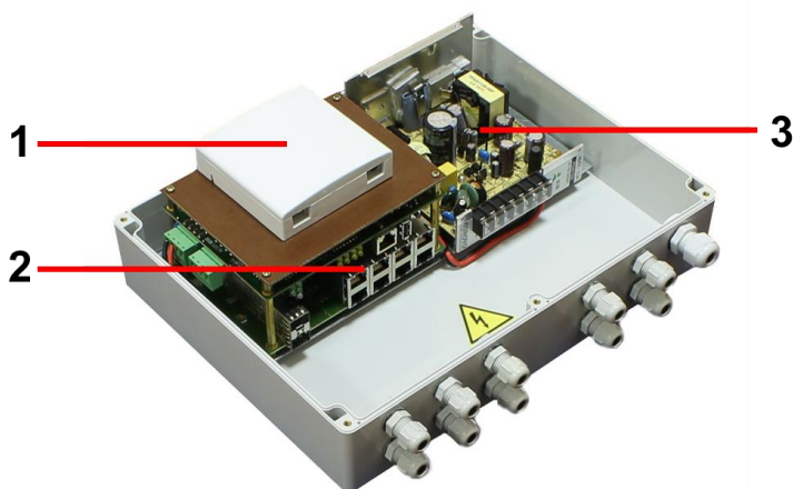
Рис.2 Уличный коммутатор SW-80802/WLC, основные элементы
