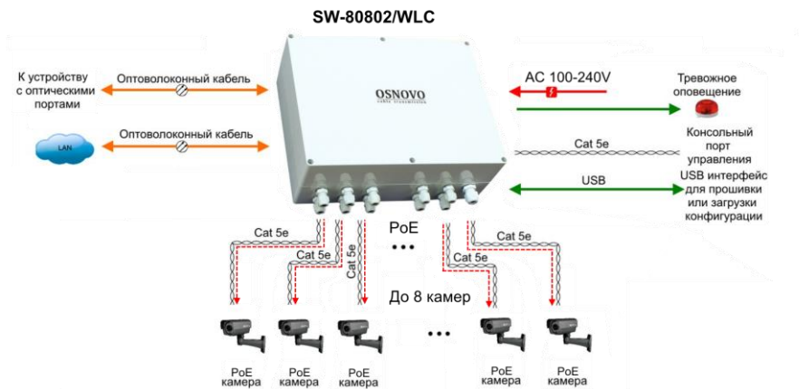
Рис.7 Типовая схема подключения коммутатора SW-80802/WLC
