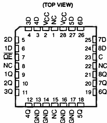
54AC11373 . . . FK PACKAGE
