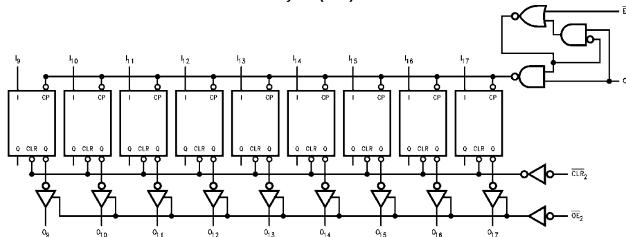
Byte 2 (9:17)
