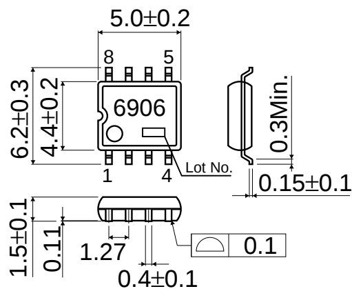
SOP 8(UNIT:mm)
