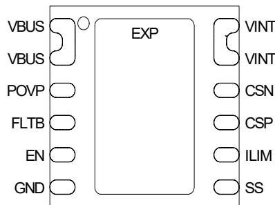
3mm x 3mm DFN-12L
