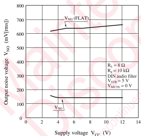
V_{\text{NO}} — V_{\text{CC}}
