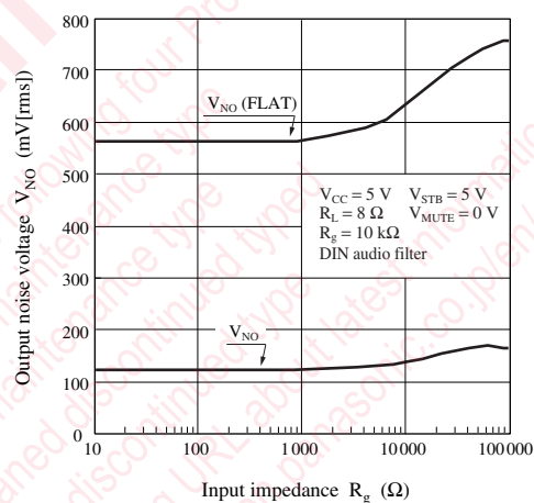
V_{\text{NO}} — R_{\text{g}}
