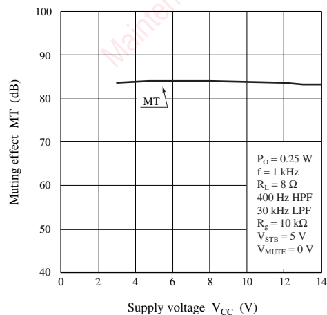
MT — V_{\text{CC}}
