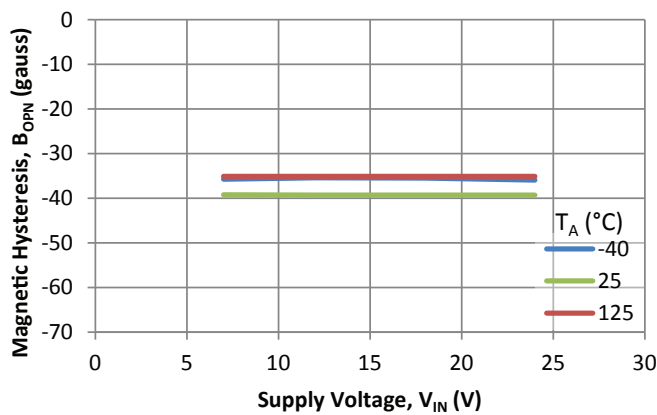
B_{OPN} vs. V_{IN}
