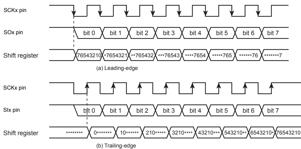
Figure 12-15 Shift Edge
