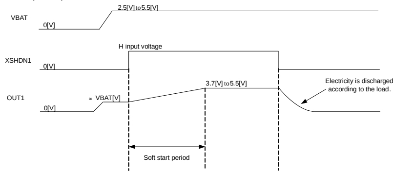
(d) PWM/PFM
