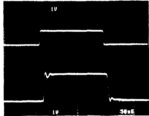
Vertical Scale: V_{IN} = 1V/Div. , V_{OUT} = 1V/Div. Horizontal Scale: 50ns/Div.
