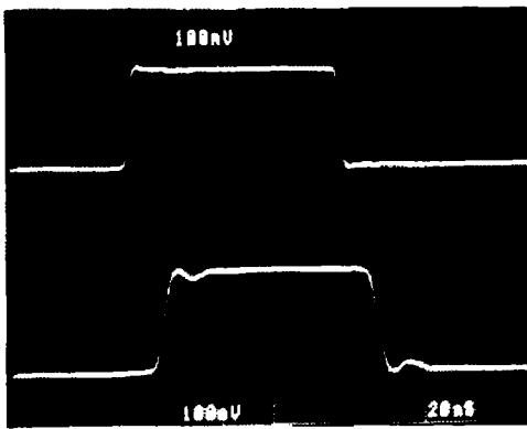
Vertical Scale: V_{IN} = 100mV/Div. , V_{OUT} = 100mV/Div. Horizontal Scale: 20ns/Div.
