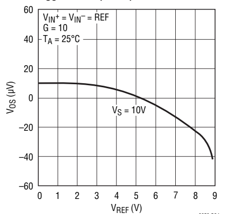
V_{OS} vs REF (Pin 5)
