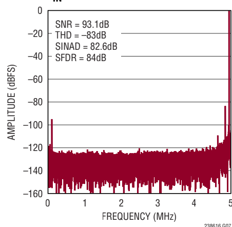
32k Point FFT f_{\text{SAMPL}} = 10\text{Mps} , f_{\text{IN}} = 5\text{MHz}
