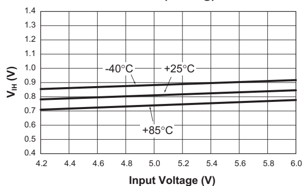
V_{IL} vs. Input Voltage EN Pin (Falling)
