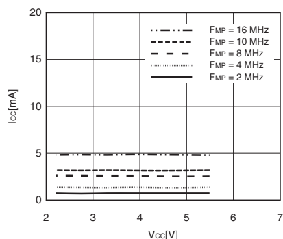
I_{CCS} - V_{CC}
