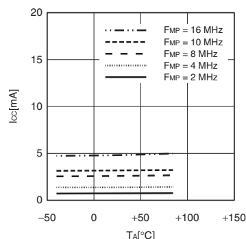
I_{CCS} - T_A
