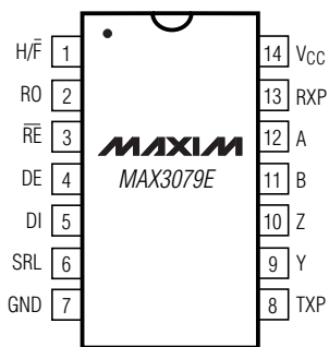
DIP/SO
