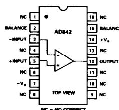
SOIC (R-16) Package
