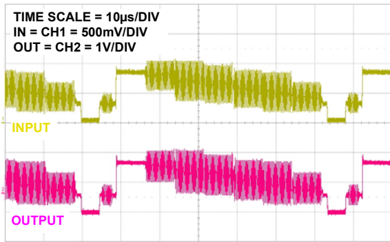
FIGURE 17. NTSC COLORBAR
