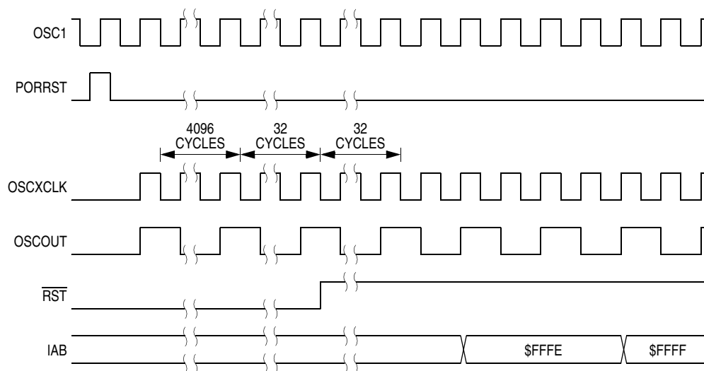
Figure 9-7. POR Recovery
