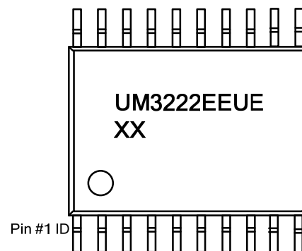
XX: Week Code UM3222EEUE TSSOP20
