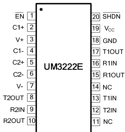
TSSOP20
