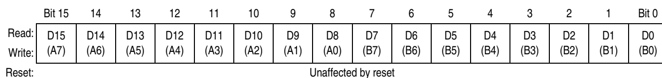
Figure 3-4. Accumulator D (D)
