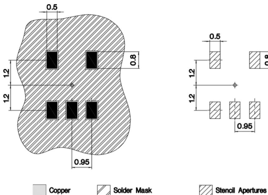
Footprint dimensions
