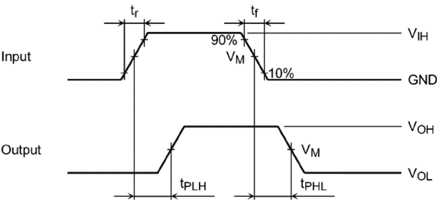
Fig. 9.7.1 t_{PLH} , t_{PHL}
