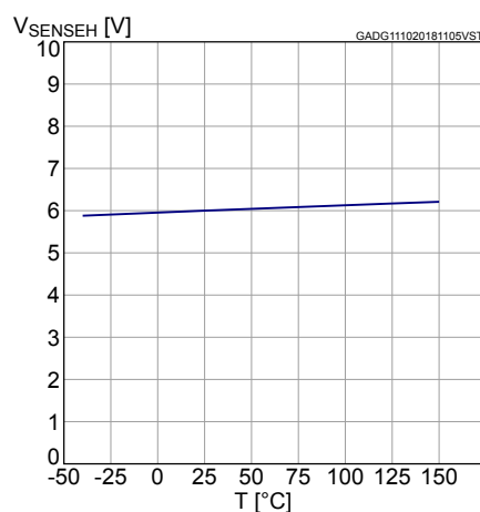
Figure 33. V_{\text{senseh}} vs. T_{\text{case}}
