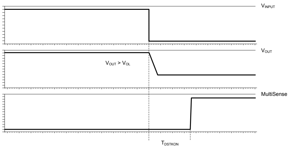
Figure 8. T_{DSTKON}
