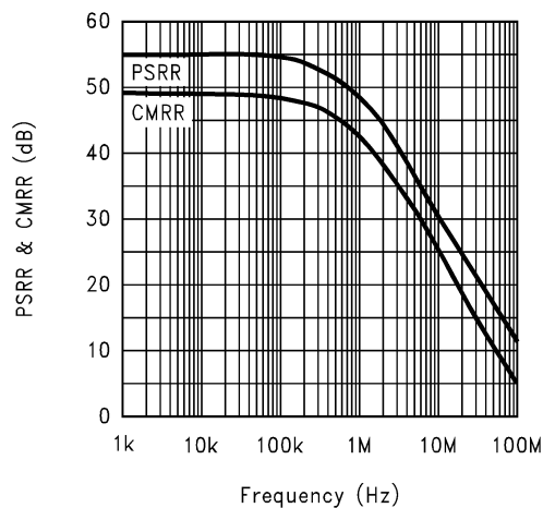
PSRR & CMRR
