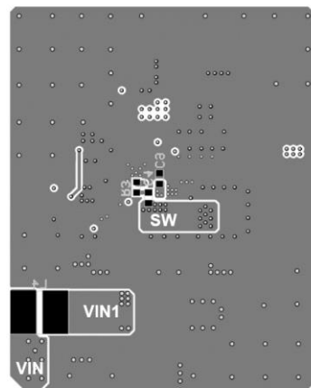
Bottom Layer
