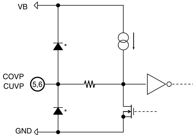
&lt;&lt;Under voltage protection block&gt;&gt;
