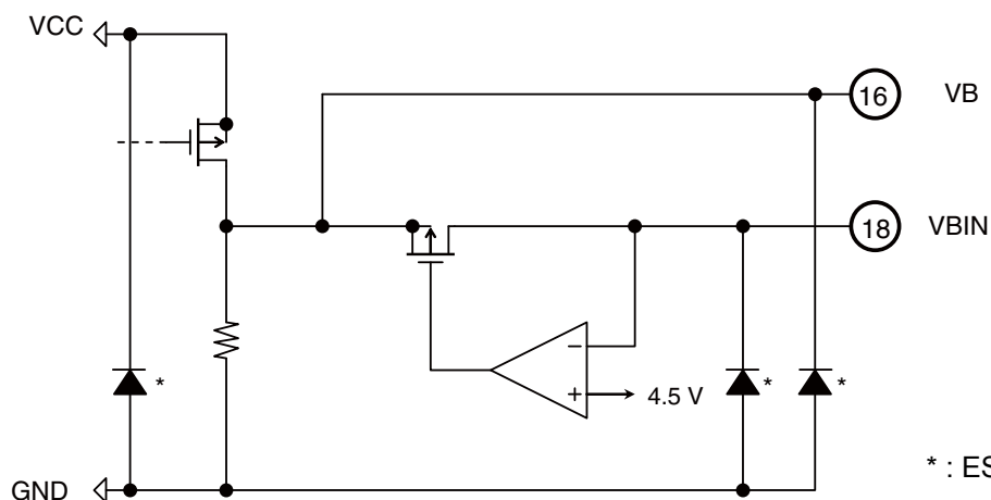
&lt;&lt;Bias voltage block&gt;&gt;
