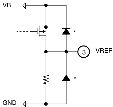
&lt;&lt;Over voltage protection block&gt;&gt;
