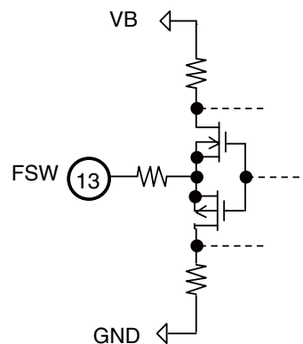
&lt;&lt;ON/OFF time generator block&gt;&gt;
