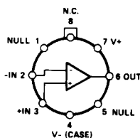
TO-99 (J-Suffix)
