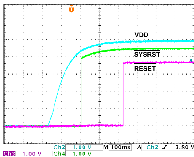
FIGURE 17. SYSRST AND RESET vs VDD (EN = VDD, 4 UVLO &gt; UVLO Vth)
