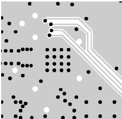
Inner Layer 3
