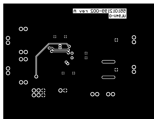
Bottom Layer
