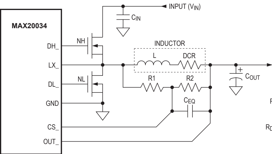
B) LOSSLESS INDUCTOR SENSING
