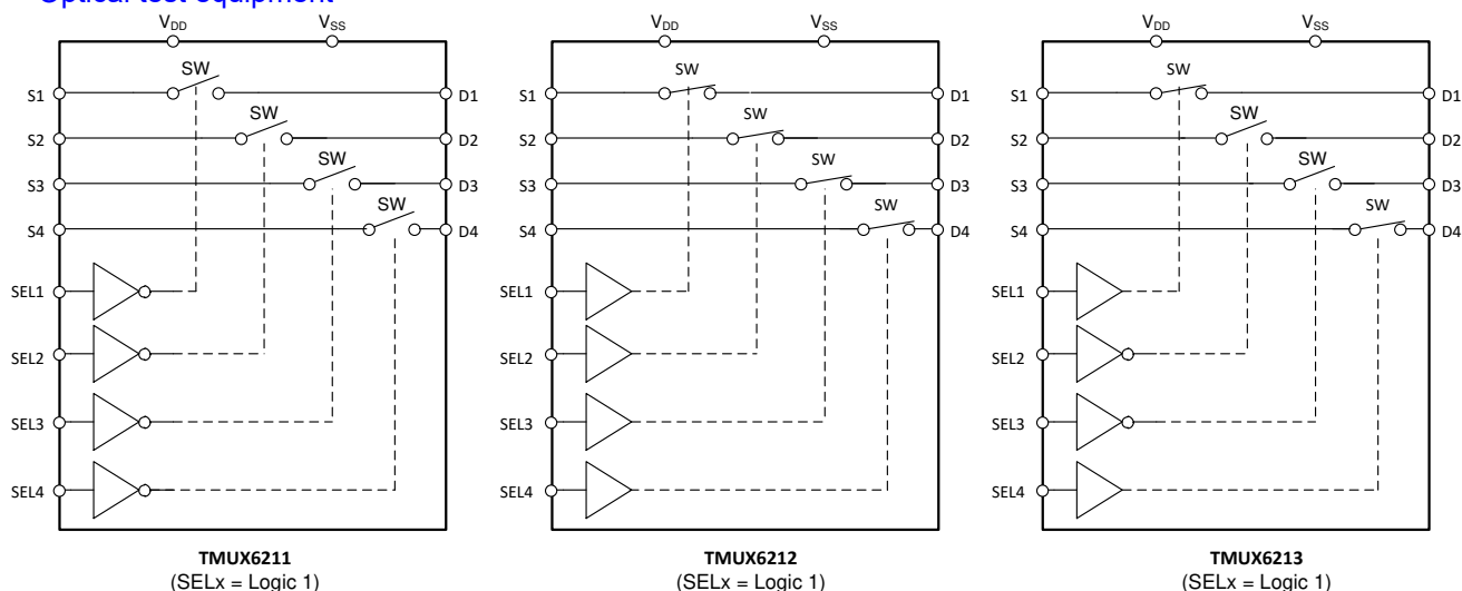
TMUX621x Block Diagrams
