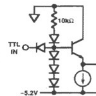
TTL Input Buffer
