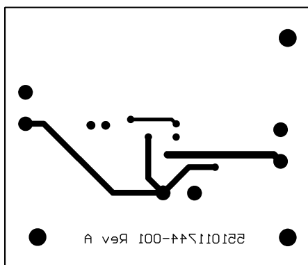
Bottom Layer
