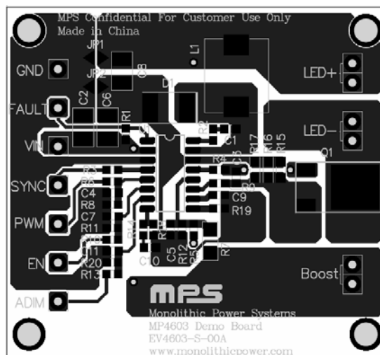
Top Layer
