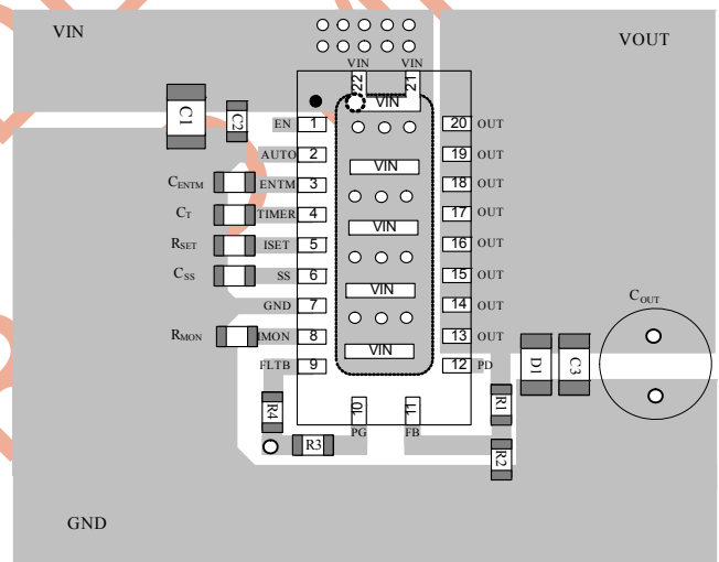
Top Layer
