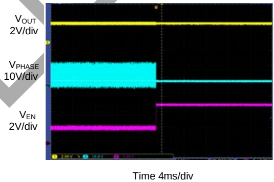
MODE Transition CCM to DEM
