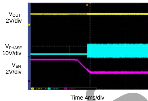
MODE Transition DEM to CCM
