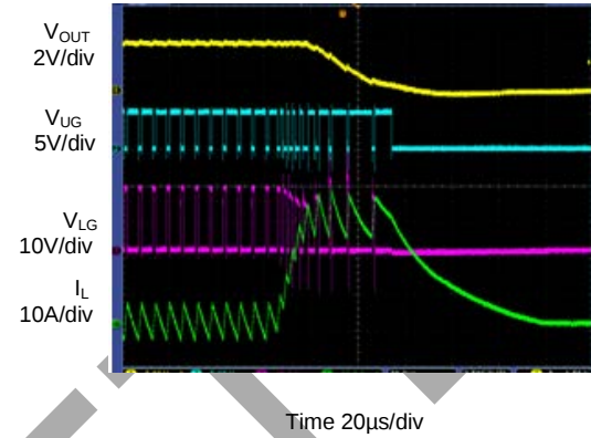
MODE Transition CCM to DEM
