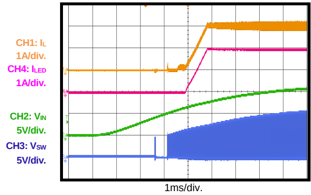
VIN Start-Up
