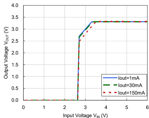
VR=3.3V
