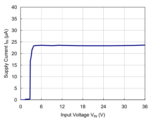
VR=3.3V
