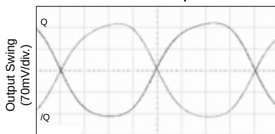
2.5GHz Output
