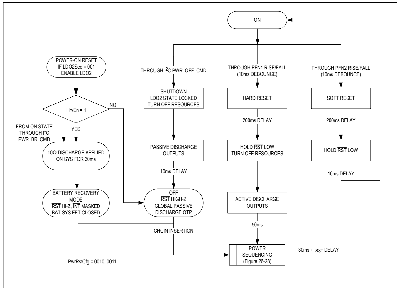
Figure 16. PwrRstCfg 0010, 0011
