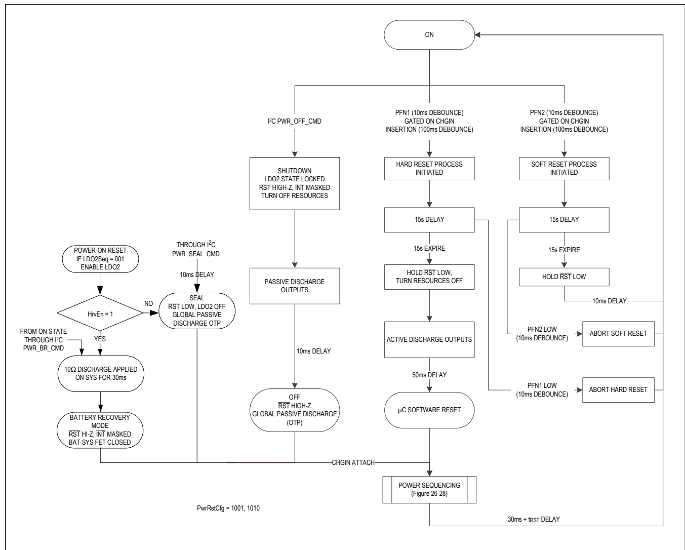
Figure 21. PwrRstCfg 1001, 1010
