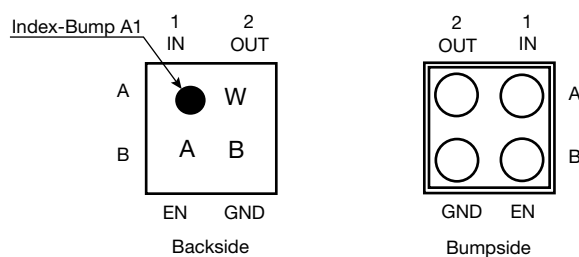
Fig. 2 - WCSP4 2 x 2 Package
