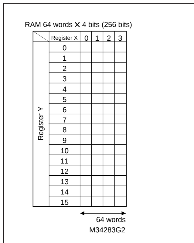
Fig. 11 RAM map
