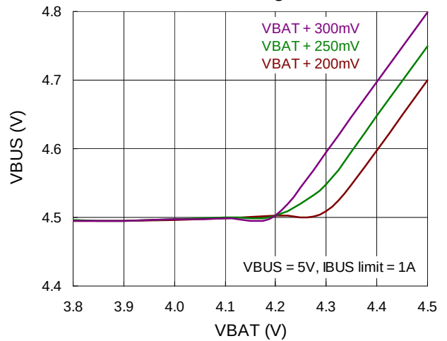
MVR Tracking VBAT
