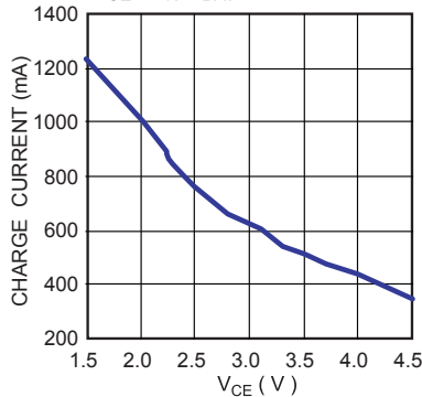
Thermal Protection ( V_{CE}=V_{IN}-V_{BAT} )
