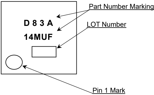
VQFN24FV4040 (TOP VIEW)
