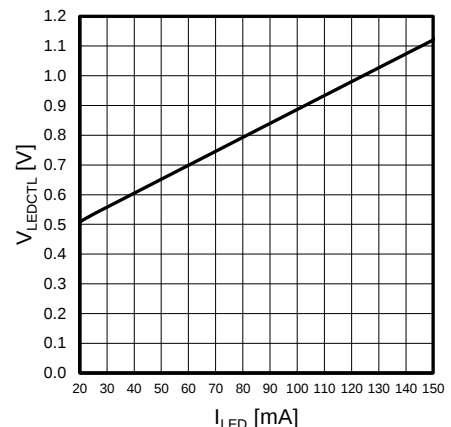
Figure 17. V_{\text{LEDCTL}} vs I_{\text{LED}}
